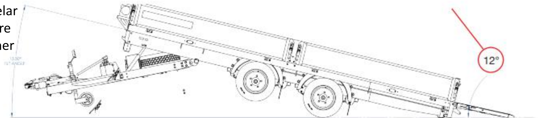
Bakramp med gasdämpare som underlättar upp och nedfällning av ramp
